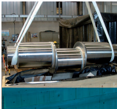
ALBERI A COLLO D'OCA
